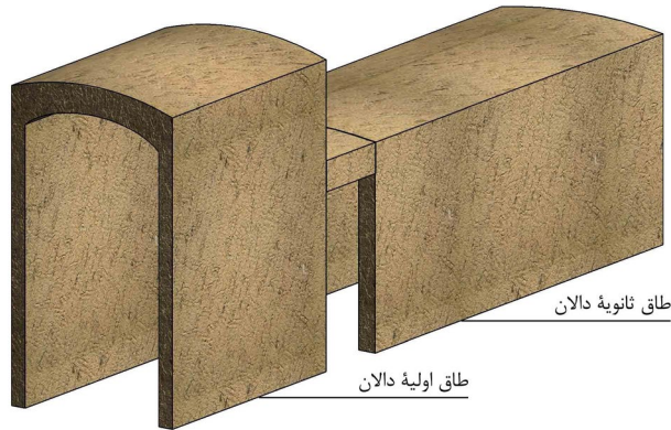
لایه قدیم و جدید طاق دالان - طاق آهنگ
