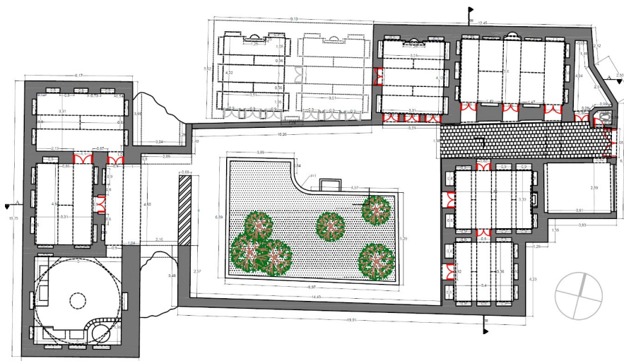
شکل ۲. پلان کنونی خانه قدیمی، مقیاس: ۱:۲۰۰، گز منبع: نگارندگان
