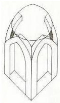
شکل ۱۲. دتایل اجرایی طاق کلمبو - منبع: مجله اثر
