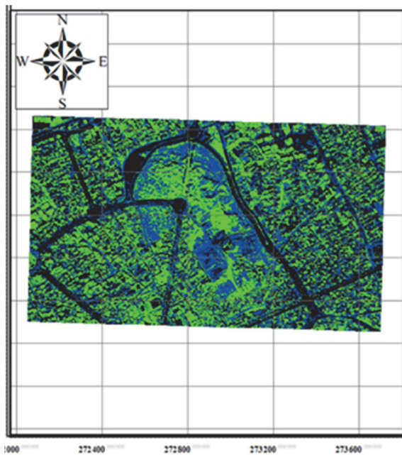
شکل ۲. نتایج طبقه‌بندی نظارت‌نشده تصویر Google Earth
