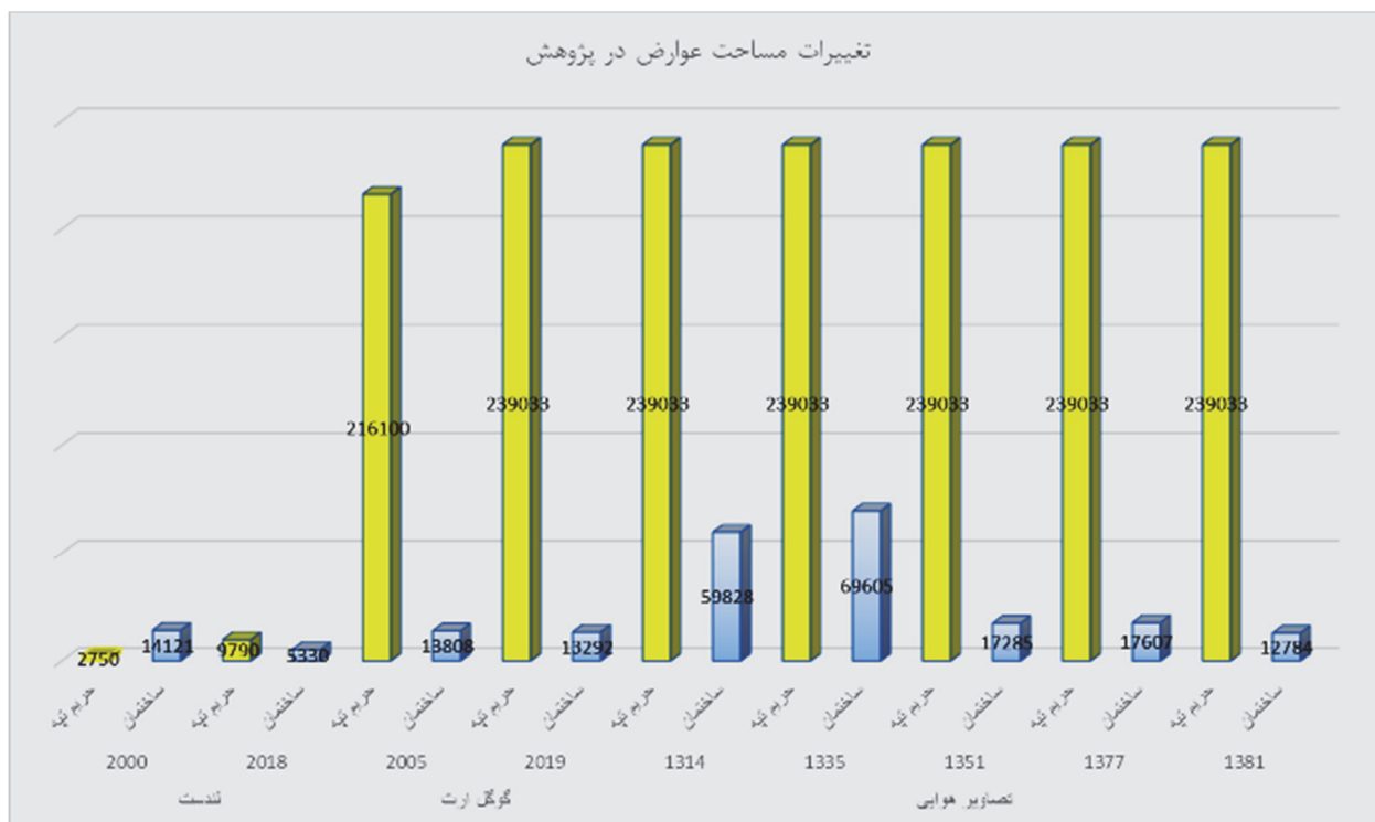
شکل ۸. نمودار ارزیابی تغییرات کاربری‌های آزمایش شده در سال‌های مورد مطالعه
