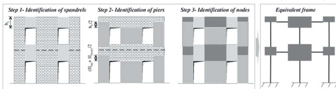
شکل ۵. نحوه مدل‌سازی یک قاب مصالح بنایی با بازشوهای مختلف به صورت قاب معادل (Lagomarsino et al., 2013)
