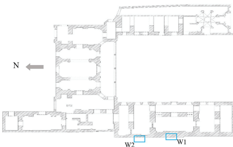
شکل ۷. محل‌های انجام تست فلت جک در ساختمان قدکی (Aminifar et al., 2022)
