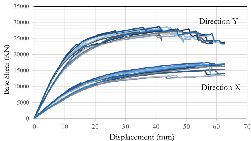
شکل ۱۱. نمودار نیرو - تغییر مکان برای هر ۲۴ حالت در شرایط بعد از استحکام بخشی
