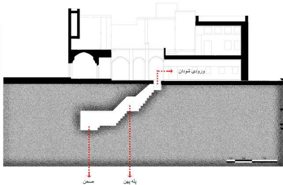
شکل ۴. ارتباط عمودی شوادان با بنای ساخته‌شده (پلان و مقطع از خانه سوزنگر) (Authors, 2022)
