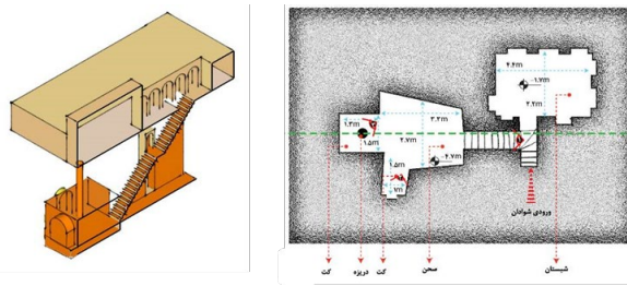
شکل ۱۸. پلان گونه منفرد شوادان (سمت راست) و برش سه‌بعدی گونه منفرد (سمت چپ) (Authors, 2022)
