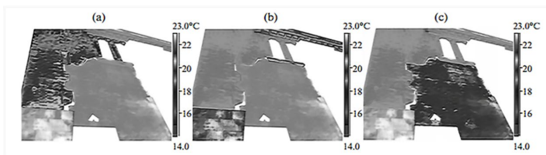
شکل ۱۲. تجزیه و تحلیل مصالح نما a. آجر، b. سنگ و c. دیوار با خاک کوبیده منبع (Lerma et al., 2018)
