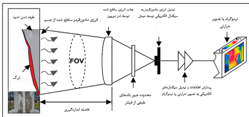
شکل ۲. نحوه عملکرد گرماسنجی مادون قرمز منبع (Jo et al., 2013)
