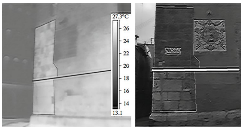
شکل ۱۱. رفتار حرارتی متفاوت سنگ در گوشه جنوب غربی ساختمان منبع (Lerma et al., 2018)
